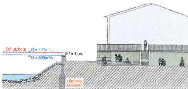
② Linksufrige Schutzmauer Höhe HQ100; Freibord mit mobilem Element bis HQ300 abgesperrt. Querschnitt im Mst. 1: 400.
